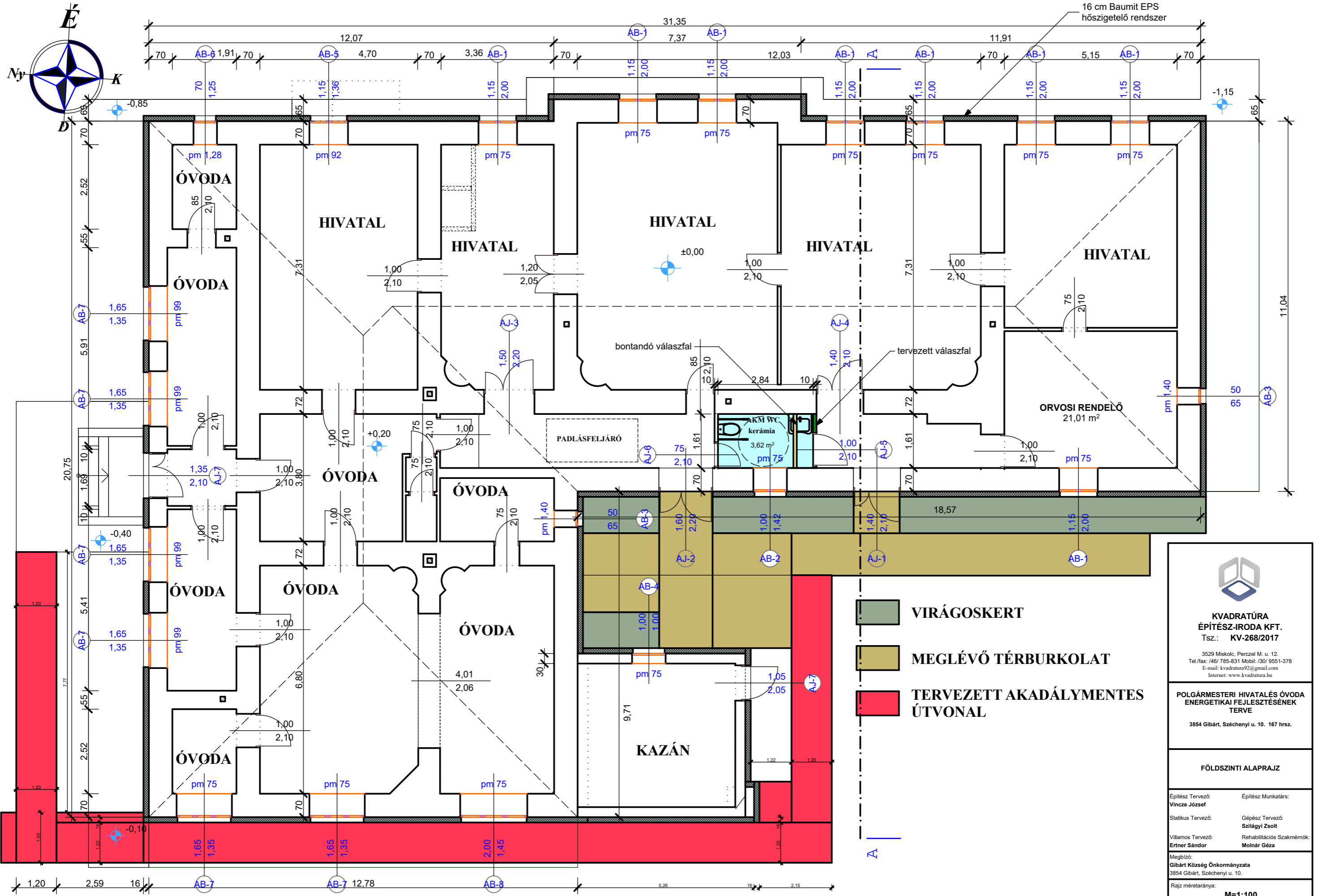
FÖLDSZINTI ALAPRAJZ M=1:100
